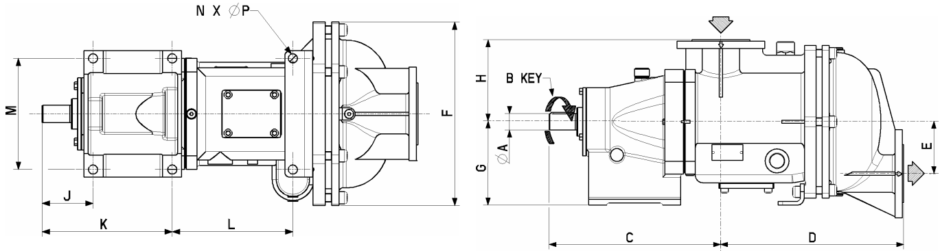
C12-A & C18-A PUMP DIMENSIONS
