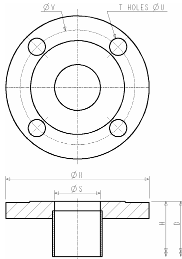
C12-A & C18-A 2 1/2" FLANGE DIMENSIONS
